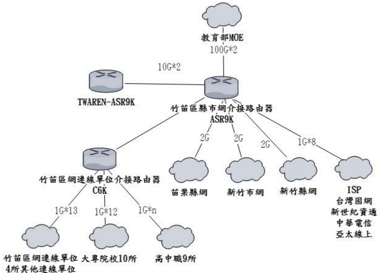
圖一：竹苗區網連線單位架構簡圖
